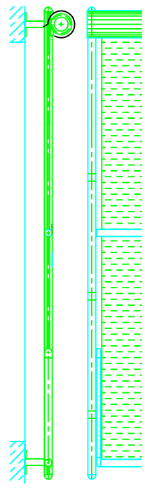
3. Version als Senkrechtmarkise Arme in Schiene eingefahren (180°)
