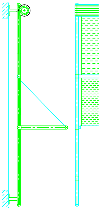
2. Version als Markisolette Ausfall der Arme 90°
